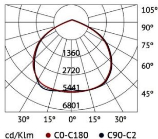
Кривая силы света
